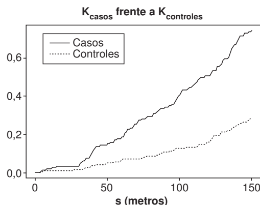
Figura 2a. Función de agregación K de Ripley para el patrón de los casos y para el de los controles.
